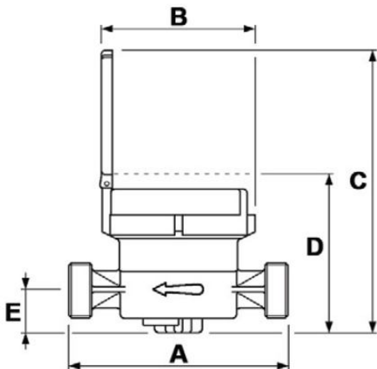
rys.1 wymiary wodomierza
